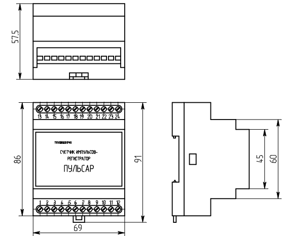
Габаритные размеры счетчика импульсов-регистратора «ПУЛЬСАР»
