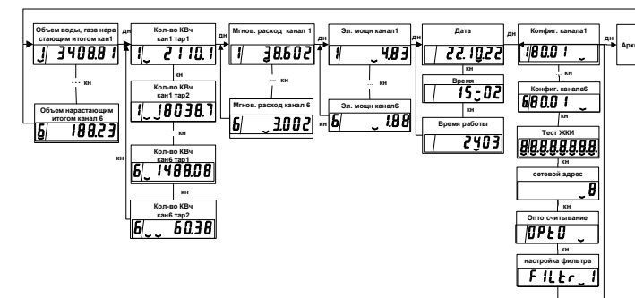
Рис. 4.2. Схема меню
