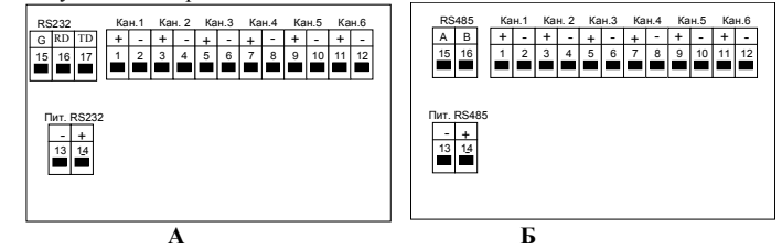
Рис. 6.2. Схема клемников платы коммутации с интерфейсом RS232 (А) и RS485 (Б)
