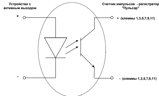
Рис. 6.1. Схема подключения устройств с активным выходом
