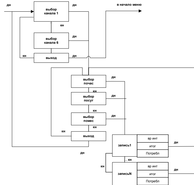
Рис. 4.3. Меню архив
