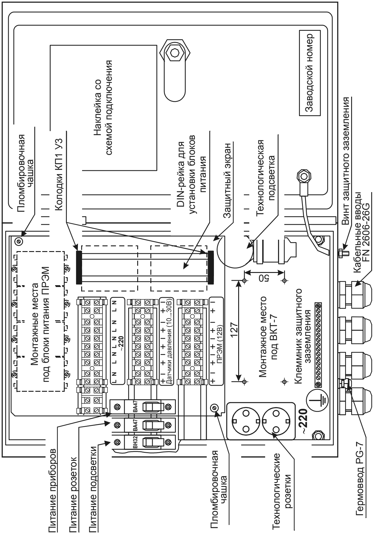
Рисунок 1 – Внешний вид монтажного шкафа ШМ7
