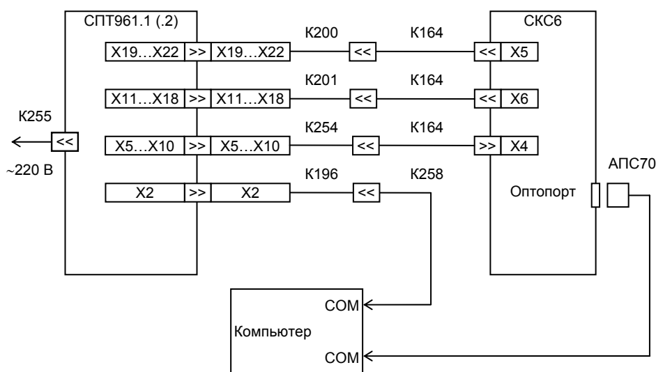
Рисунок 5.1 Схема проверки
