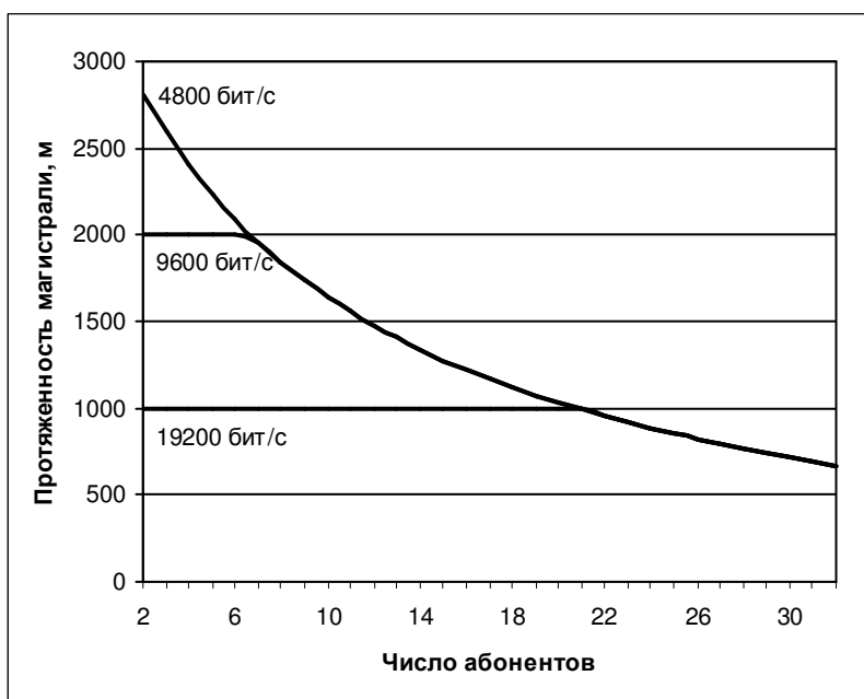
Рисунок 5 – Протяженность магистрали при ее прокладке кабелем UTP (FTP) категории 5
