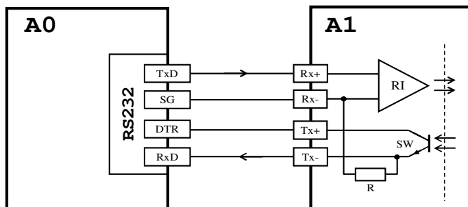
A0 – ведущий абонент с интерфейсом RS232; A1 – ведомый абонент; RI – приемный буфер; SW – передающий ключ; R – балластное сопротивление передатчика
